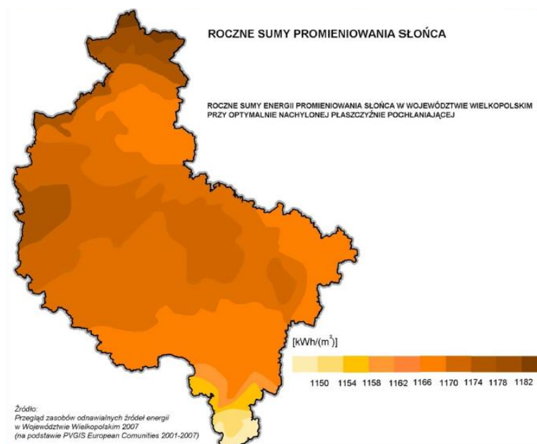
Rysunek 8. Roczne sumy promieniowania słonecznego dla Wielkopolski
