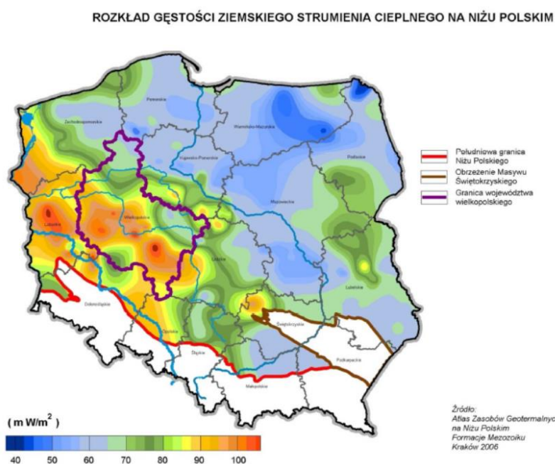
Rysunek 9. Mapa gęstości ziemskiego strumienia ciepłego dla obszaru polski Źródło: Energetyka odnawialna w Wielkopolsce uwarunkowania rozwoju, Poznań 2012
