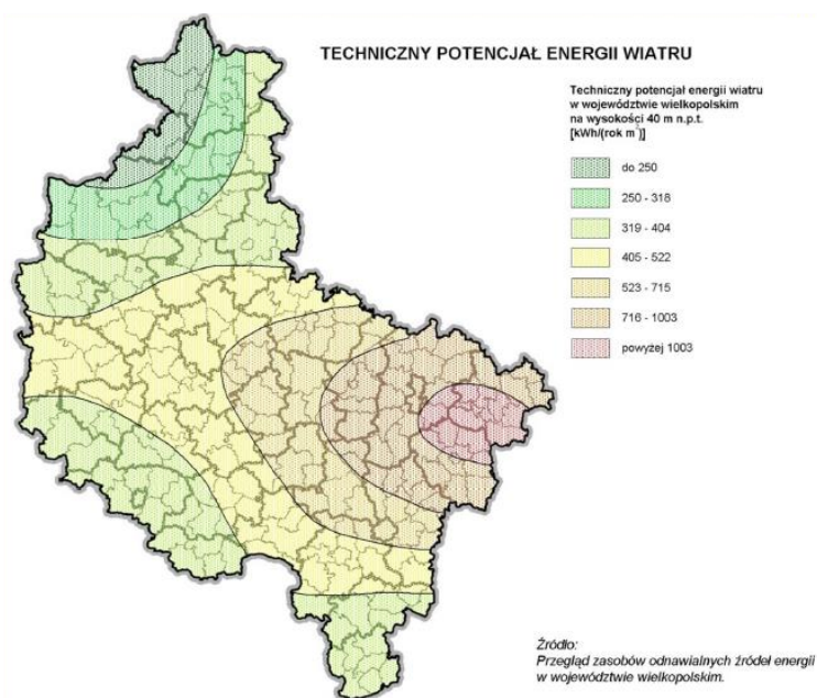
Rysunek 7. Techniczny potencjał energii wiatru dla Wielkopolski i poszczególnych powiatów
